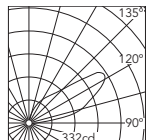
Luminous flux luminaire 1440 lm
