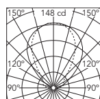
Luminous flux luminaire 269 lm
