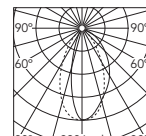
Luminous flux luminaire 2204 lm
