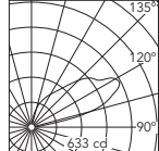
Luminous flux luminaire 2177 lm
