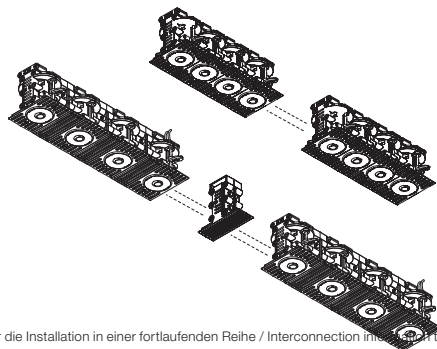
Verbindungsdetail für die Installation in einer fortlaufenden Reihe / Interconnection in order to build a continuous line
