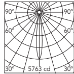
Luminous flux luminaire 403 lm
